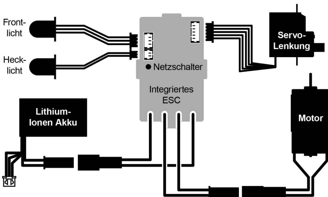
Anschlussplan der elektronischen Ausrüstung
