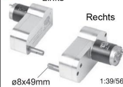
CNC Antriebsgetriebe (Craftsman-Serie)
