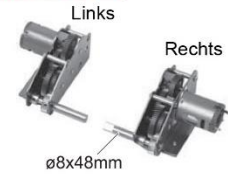
Antriebsbox Ultimate Edition (Vollwellenlager, Stahlgetriebe)
