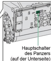
Hauptschalter des Panzers (auf der Unterseite)
