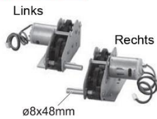
Metall-Getriebeantriebsgehäuse (A: Zinklegierung, B: Stahlgetriebebehälter)
