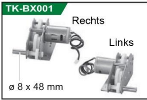
Antriebsgetriebe (Kunststoffgetriebe)
