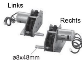
Metall-Getriebeantriebsgehäuse (A: Zinklegierung, B: Stahlgetriebebehälter)
