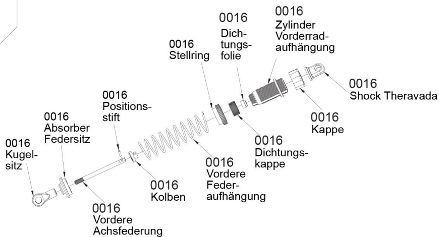
0016 Vorderradaufhängung
